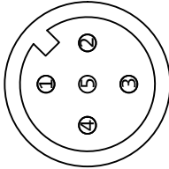
LHM3 AI1 - AI3: Analog Inputs
