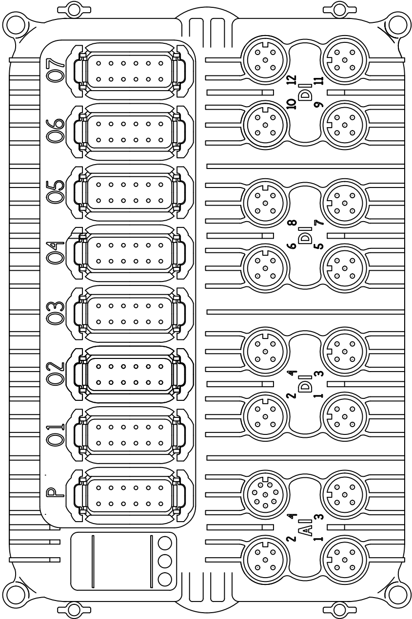
LHM3 AI4: Analog Inputs
